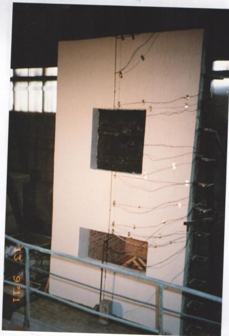
Рис.5.1. Общий вид перед огневыми испытаниями смонтированного на фрагменте железобетонной стены образца системы фасадной теплоизоляционной композиционной «ТЕРМОХА-УС».
